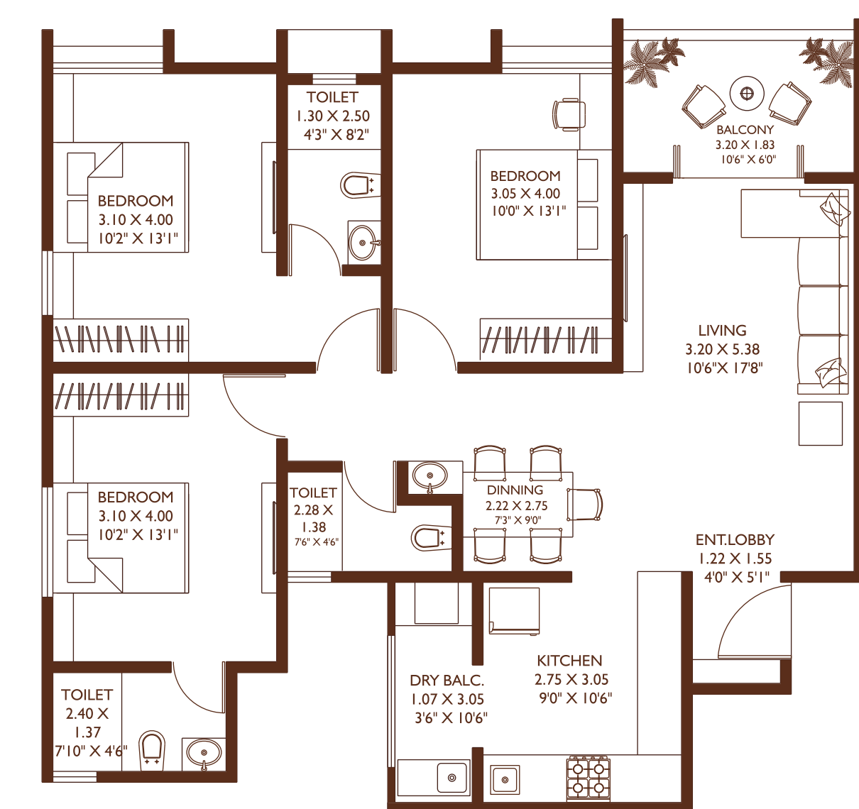
3BHK - Type 1
