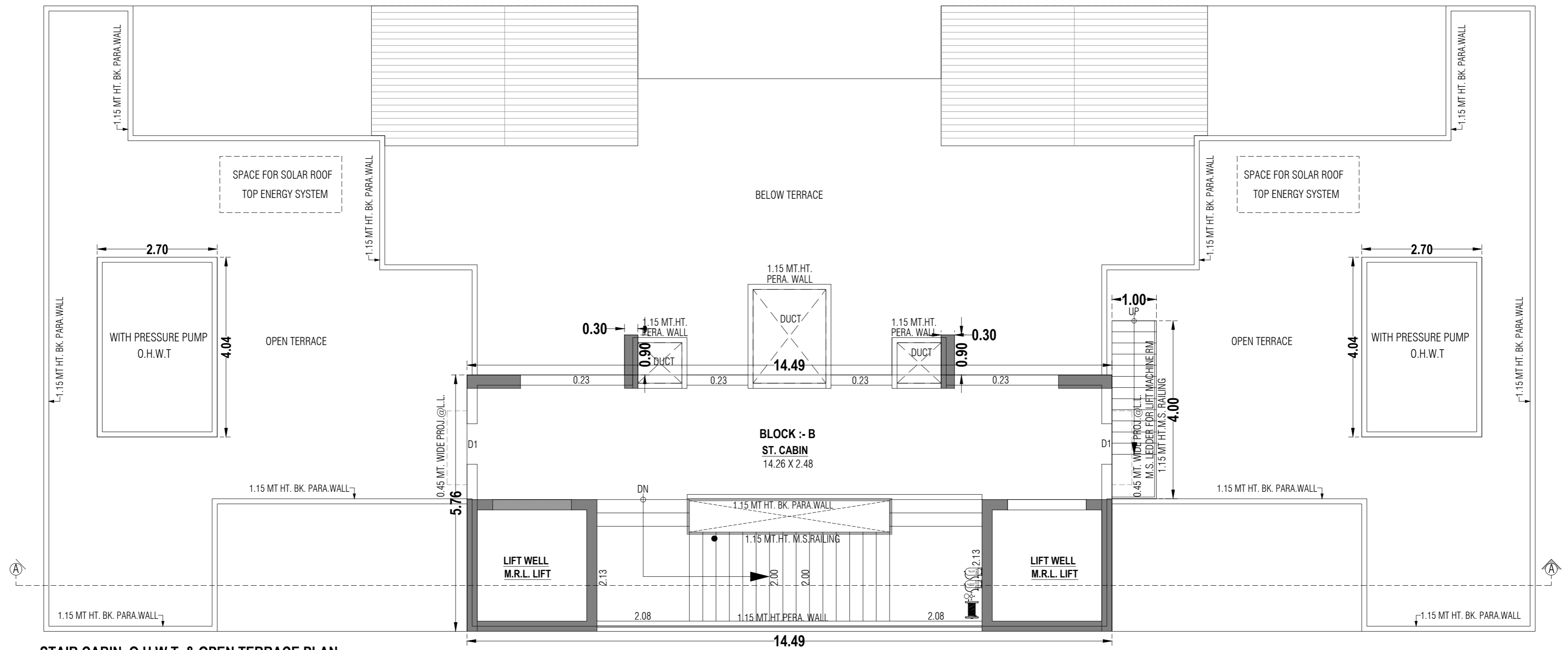
STAIR CABIN, O.H.W.T. & OPEN TERRACE PLAN
